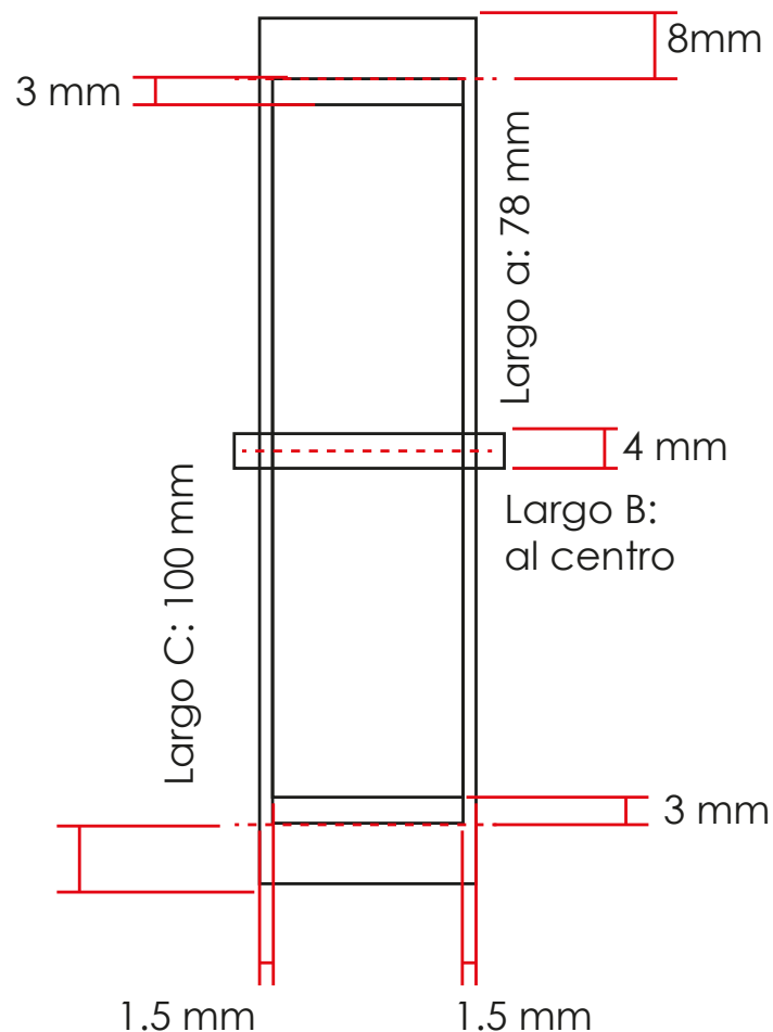
Estructura de una etiqueta bordada EJEMPLO ETIQUETA DE 100mm x 25 mm
